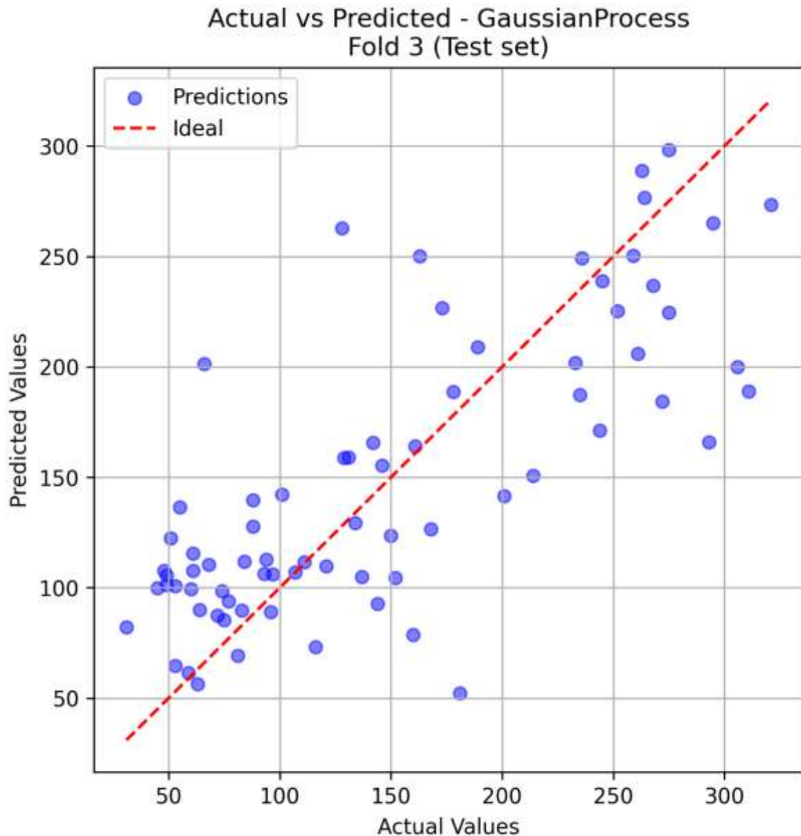
Εικόνα 2: Αποτελέσματα Actual vs Predicted για το μοντέλο Gaussian Process Regression
