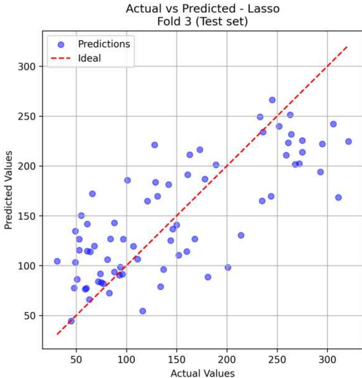
Εικόνα 4: Αποτελέσματα Actual vs Predicted για το μοντέλο Lasso
