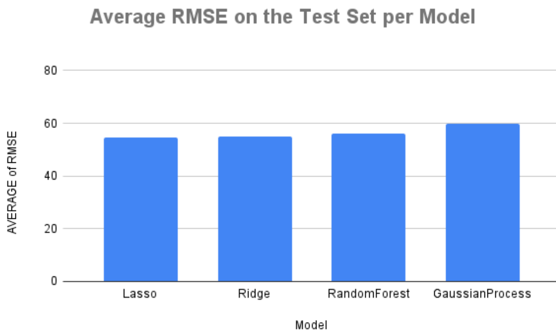
Εικόνα 5: Μέσο RMSE στο σύνολο ελέγχου (Test Set) για τα τέσσερα μοντέλα παλινδρόμησης.
