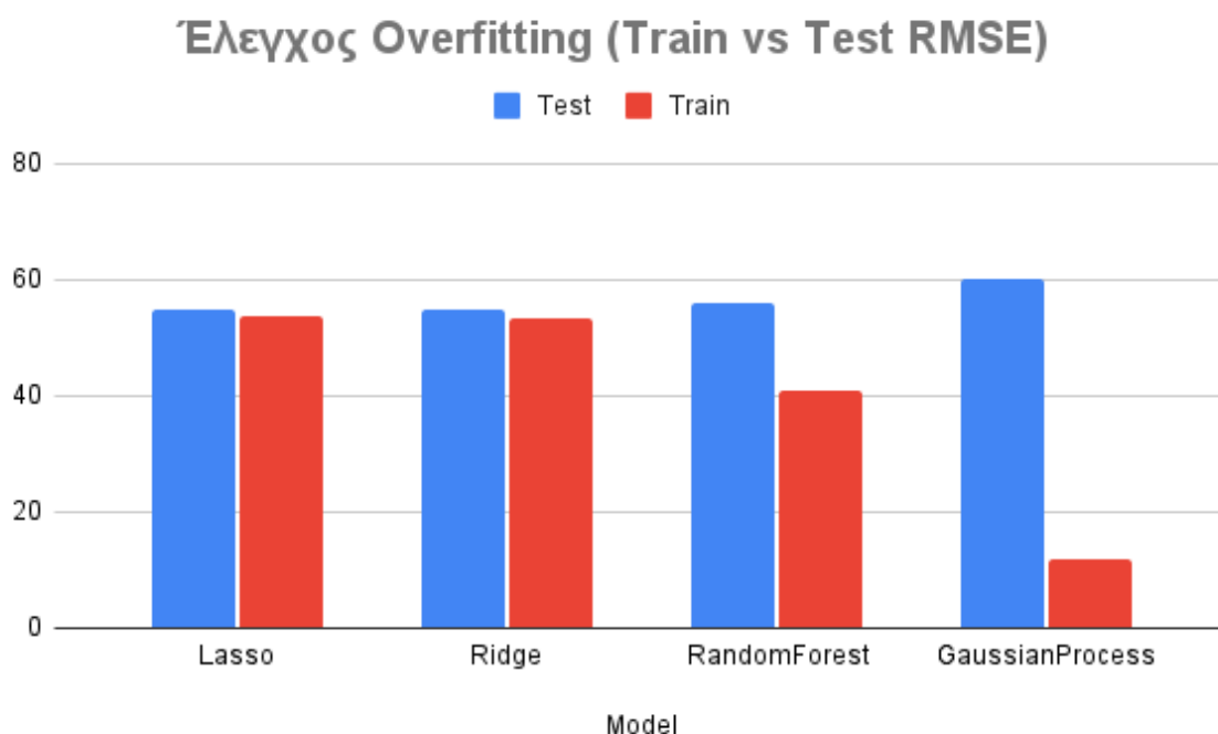
Εικόνα 8: Έλεγχος Υπερ-εκπαίδευσης (Overfitting) – Σύγκριση RMSE μεταξύ συνόλων Εκπαίδευσης (Train) και Ελέγχου (Test).
