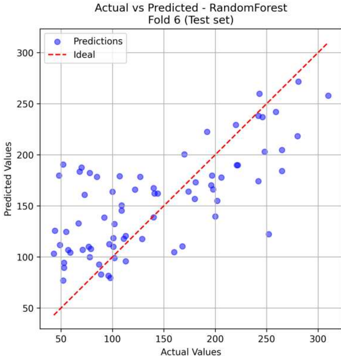
Εικόνα 1: Αποτελέσματα Actual vs Predicted για το μοντέλο Random Forest
