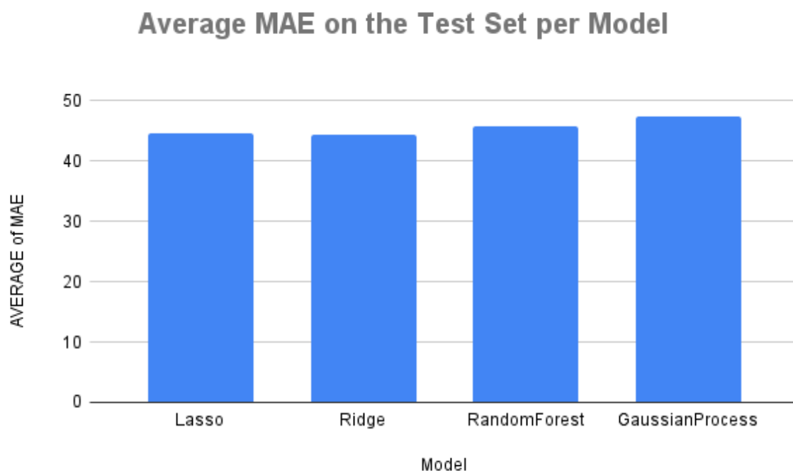
Εικόνα 6: Μέσο MAE στο σύνολο ελέγχου (Test Set) για τα τέσσερα μοντέλα παλινδρόμησης.
