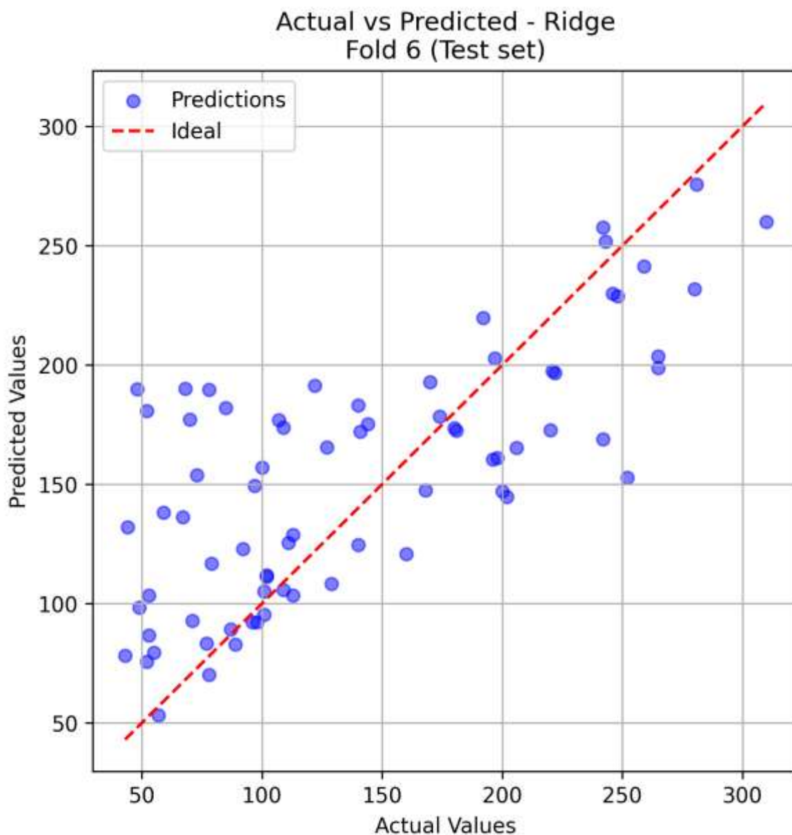
Εικόνα 3: Αποτελέσματα Actual vs Predicted για το μοντέλο Ridge Regression
