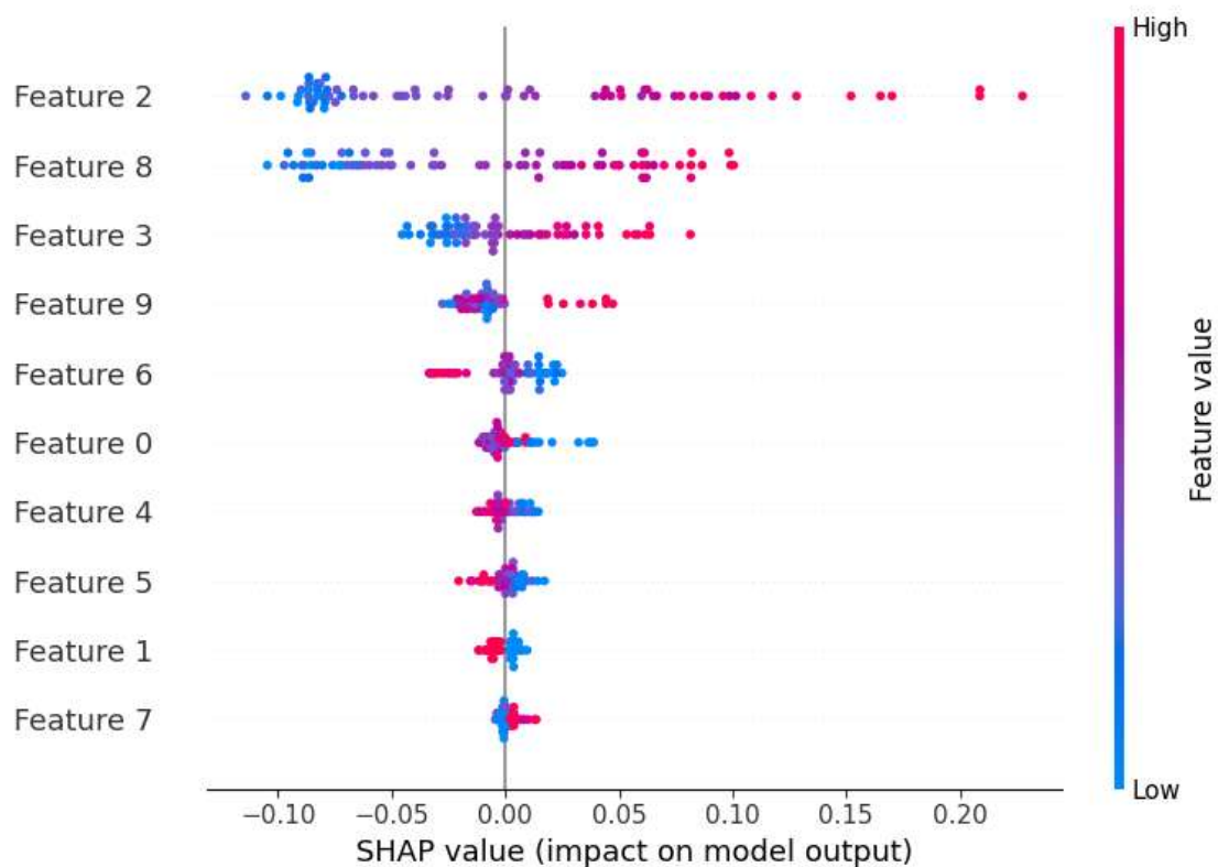
Εικόνα 9: Διάγραμμα SHAP Summary – Ιεράρχηση της επιδρασιμότητας των κλινικών χαρακτηριστικών στο μοντέλο Random Forest.
